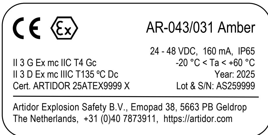
Beispiel eines Etiketts für die AR-043 Signalleuchte
