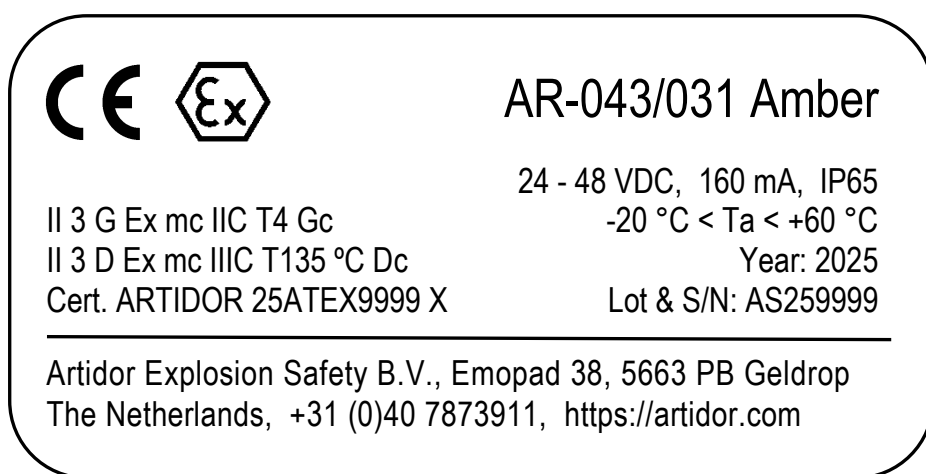
Voorbeeld van een label van het AR-043 signaallicht
