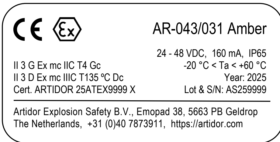
Exemple d'étiquette d'un avertisseur lumineux à LED antidéflagrant AR-043
